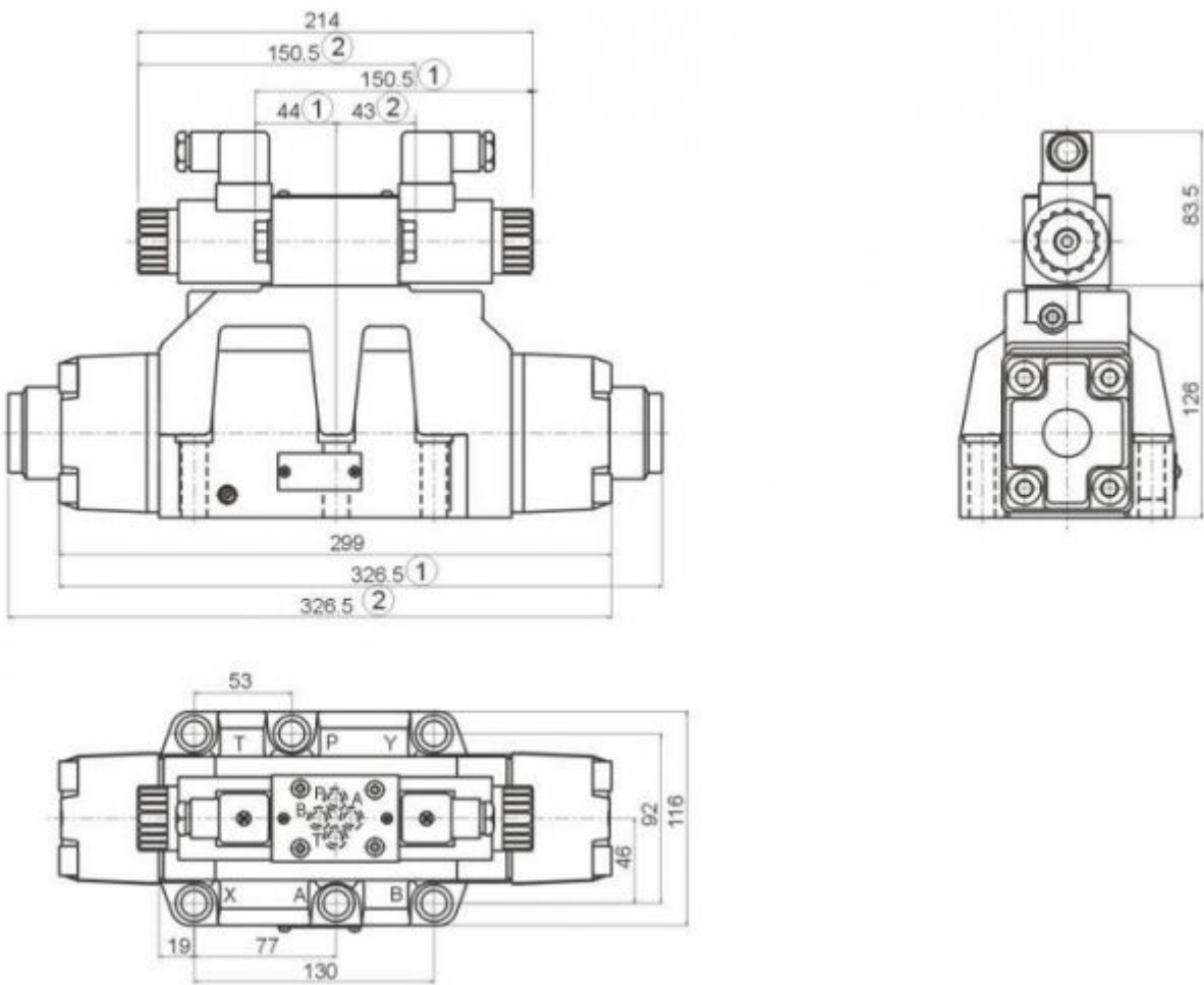
Габаритные и присоединительные размеры гидрораспределителей 1P203:
